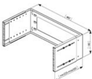
Настенный кронштейн
